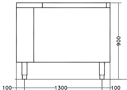
Fronte
